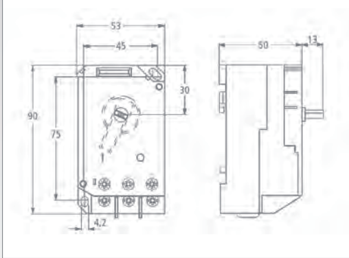
Motorschutzschalter OKN
