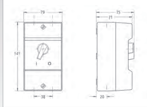
Gehäuse H
