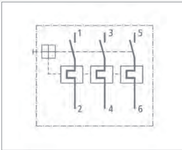
Motorschutzschalter OKN
