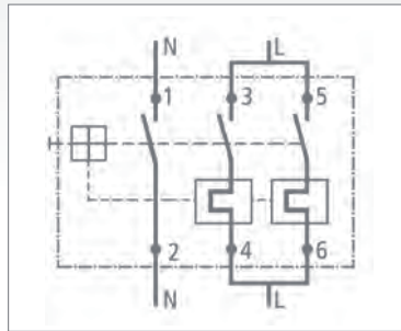
Motorschutzschalter OKN 30 u. OKN 37 (2-pol.)
