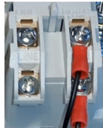
Anschluss des Zählermoduls an die Klemmen MOTOR / MOTOR
